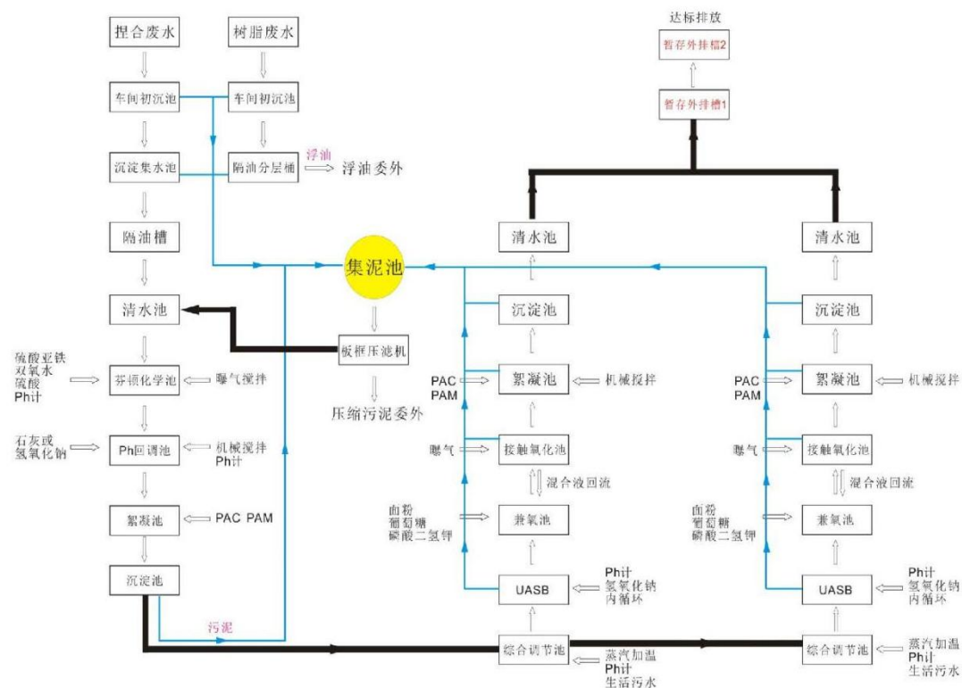
图 4.2 废水处理工艺流程图
