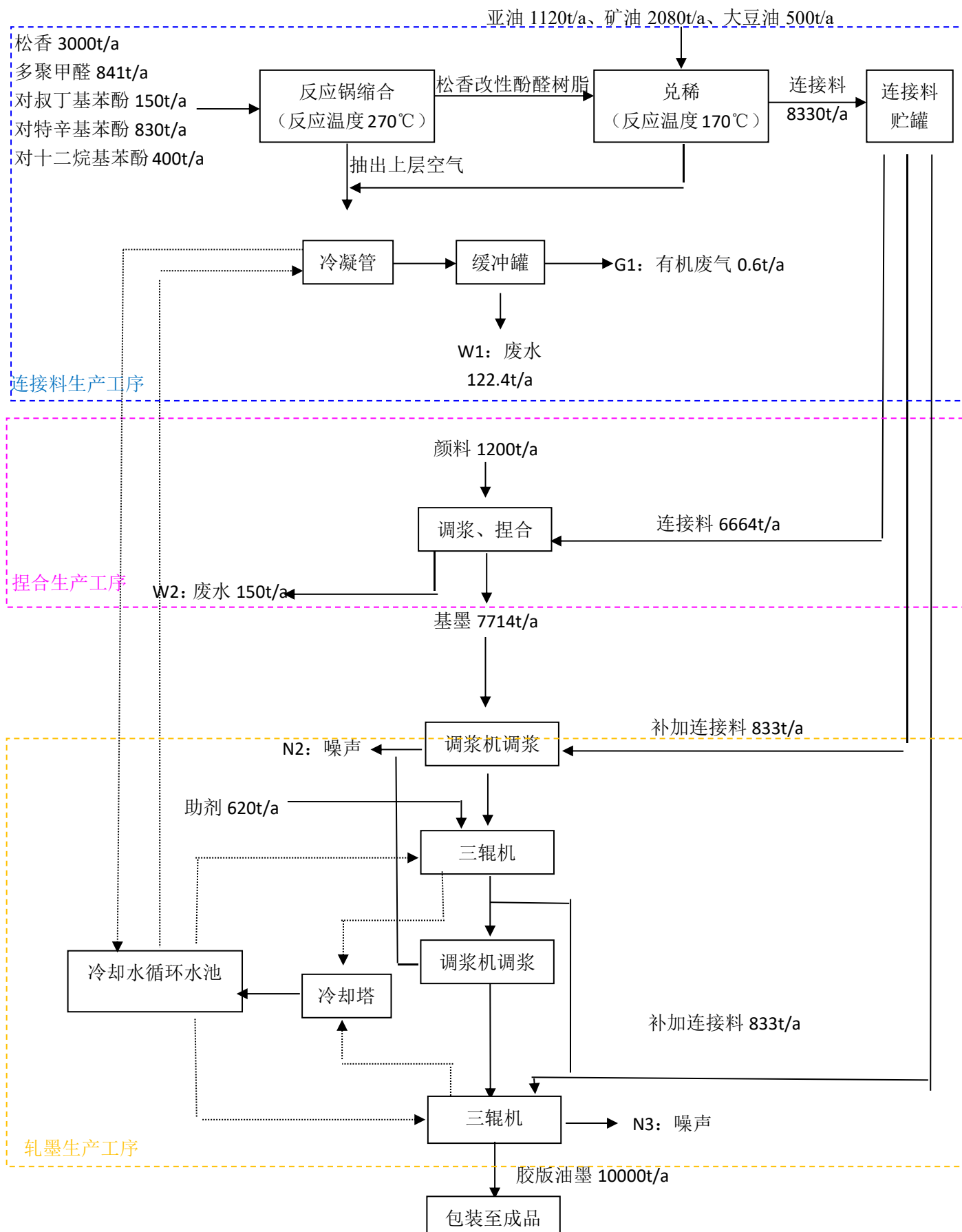
图 4.1 生产工艺流程及排污环节
